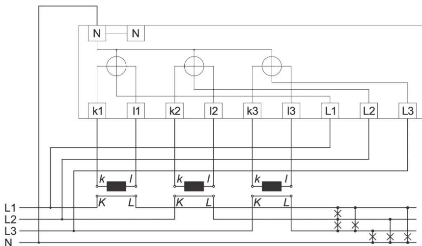
Anschlussbild Wandlerzähler SINUS 5/1 SL
